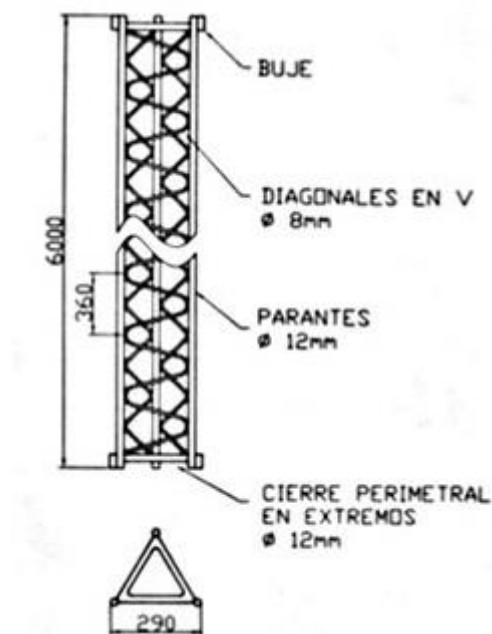
Ilustración 30 - Descripción de la torre -
