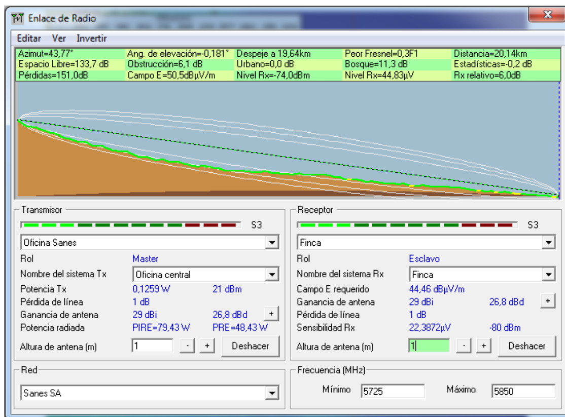
Ilustración 28 - Línea de vista entre la Oficina Central y la Finca 26 .
