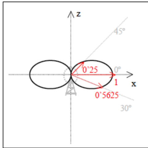
Ilustración 17 - Radiación de una Antena Omnidireccional 16 -
