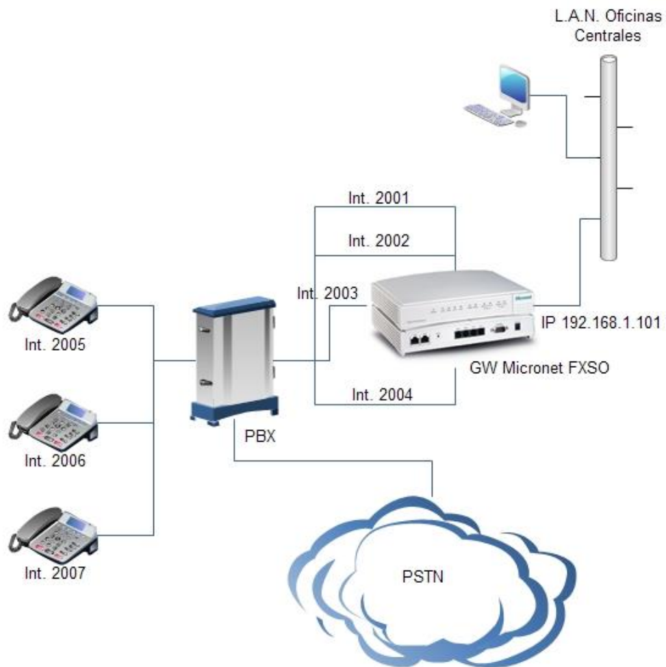
Ilustración 44 - Conexión física del GW Ip en la oficina central 44 .
