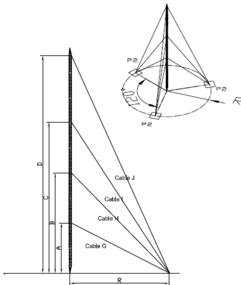
Ilustración 20 - Anclaje de las riendas -
