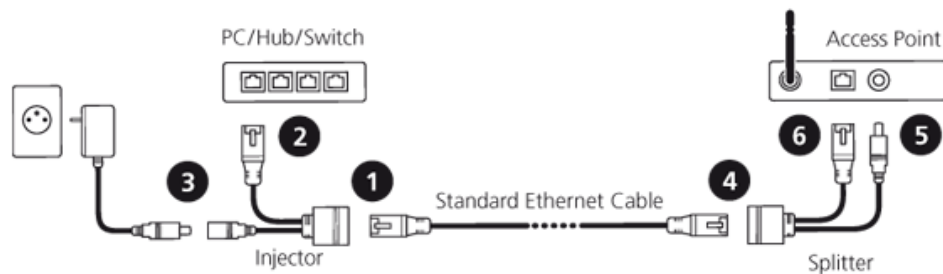
Ilustración 12 - Conexionado PoE 11 -
