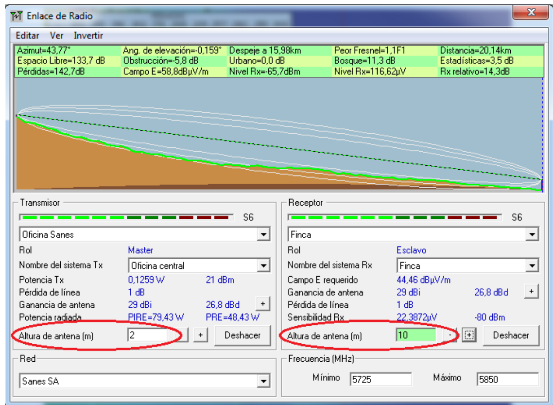
Ilustración 29 - Despeje de la 1ª zona de fresnel 27 .
