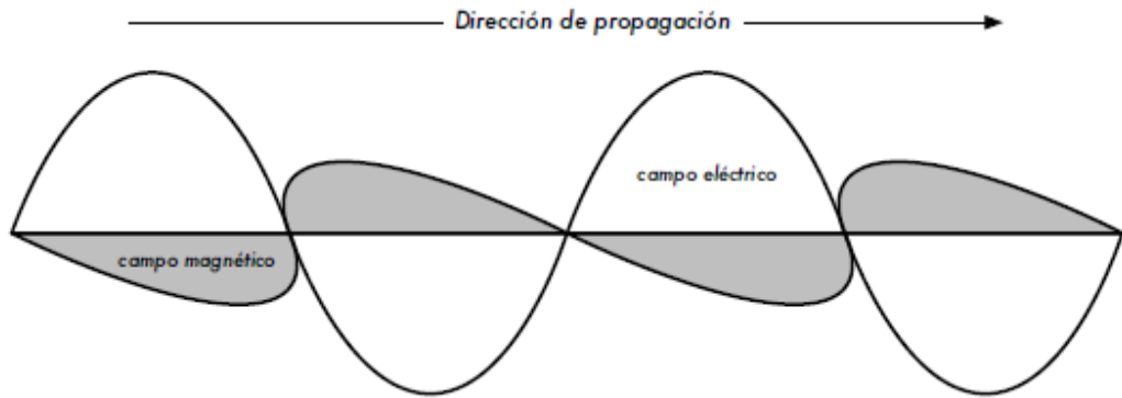
Ilustración 5 - El campo eléctrico y el campo magnético de una onda electromagnética 5 -
