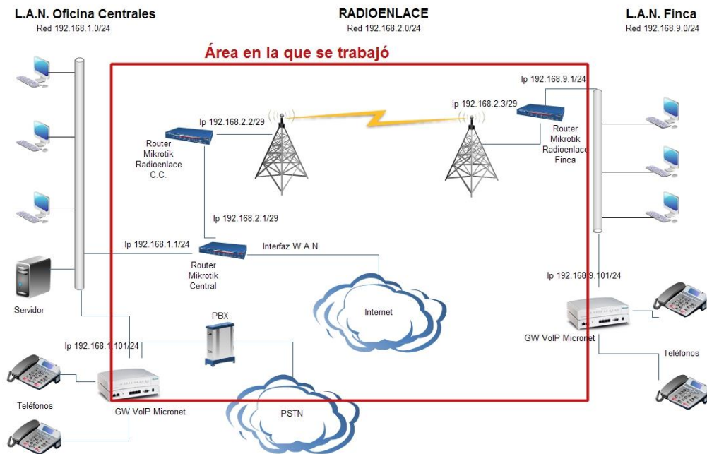
Ilustración 25 – Nuevo diseño de la red de Sanes S.A. 23 .
