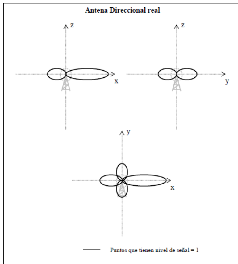
Ilustración 18 - Antena Direccional 17 -
