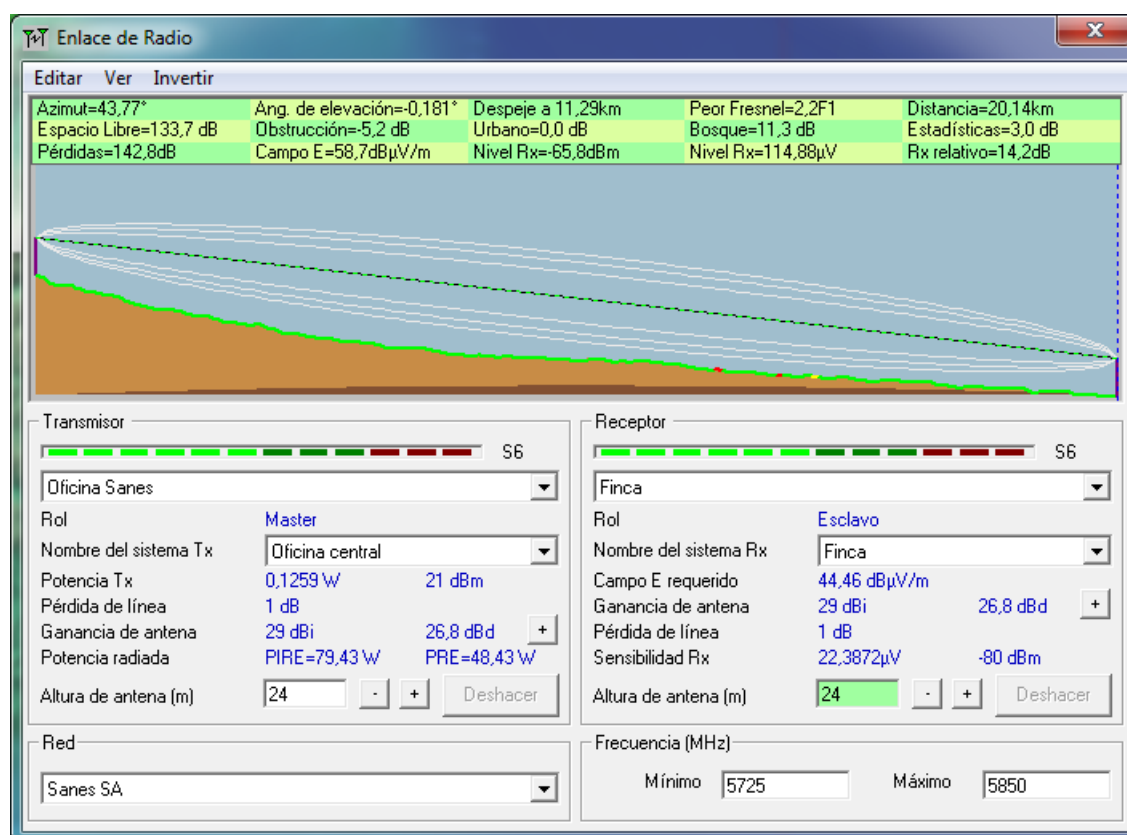
Ilustración 38 - Enlace de Radio 35 -
