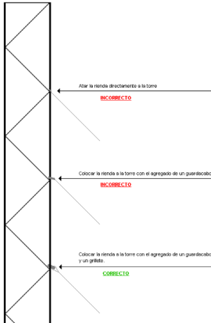
Ilustración 21 - Correcta instalación de la rienda sobre la torre - 19
