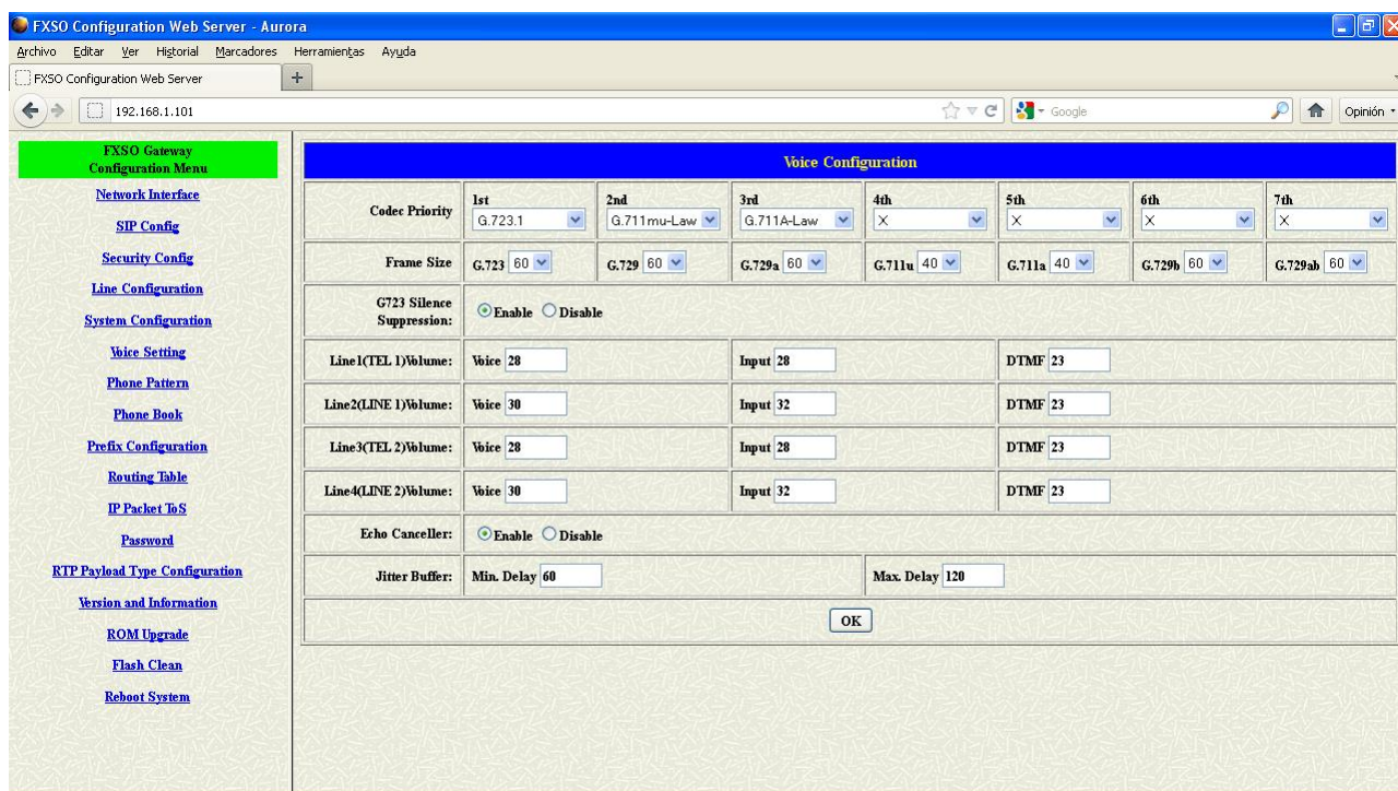
Ilustración 51 - Configuración de la voz del GW Ip 51 .
