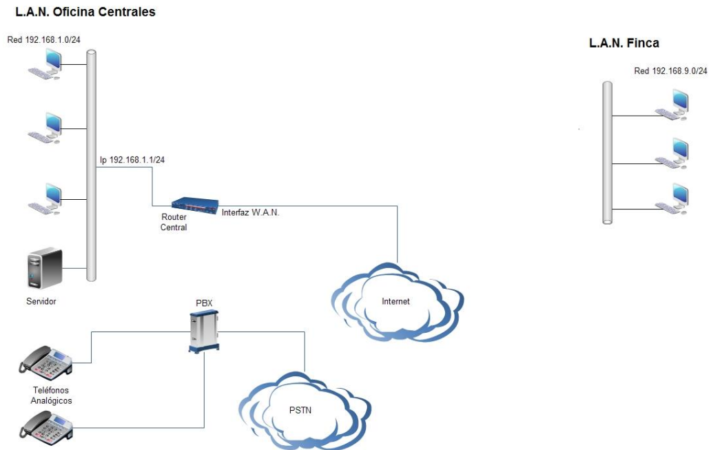
Ilustración 24 - Red de Sanes S.A. actual 22 .
