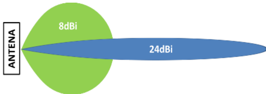
Ilustración 8 - Relación entre distancia y ganancia de una antena. - 7
