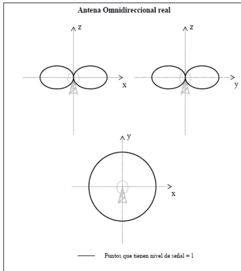
Ilustración 16 - Antena Omnidireccional Real 15 -
