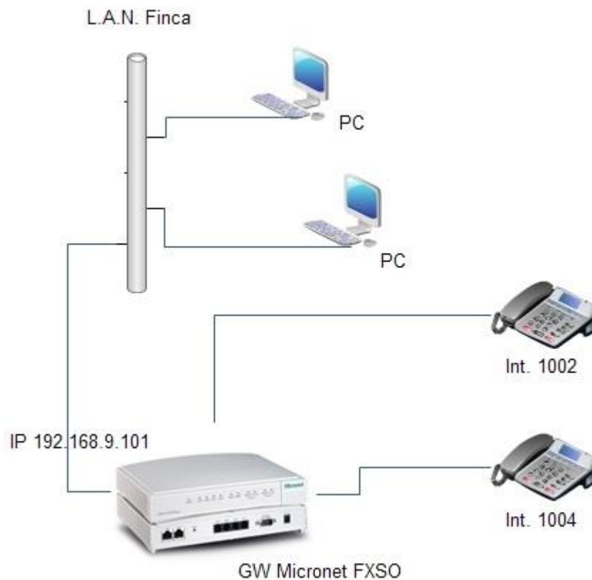
Ilustración 45 - Conexionado físico del GW Ip en la finca 45 .
