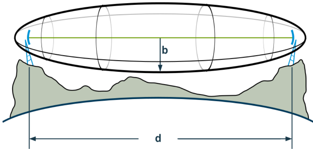
Ilustración 13 - Lóbulo de zona Fresnel de una Señal entre 2 antenas 12 .
