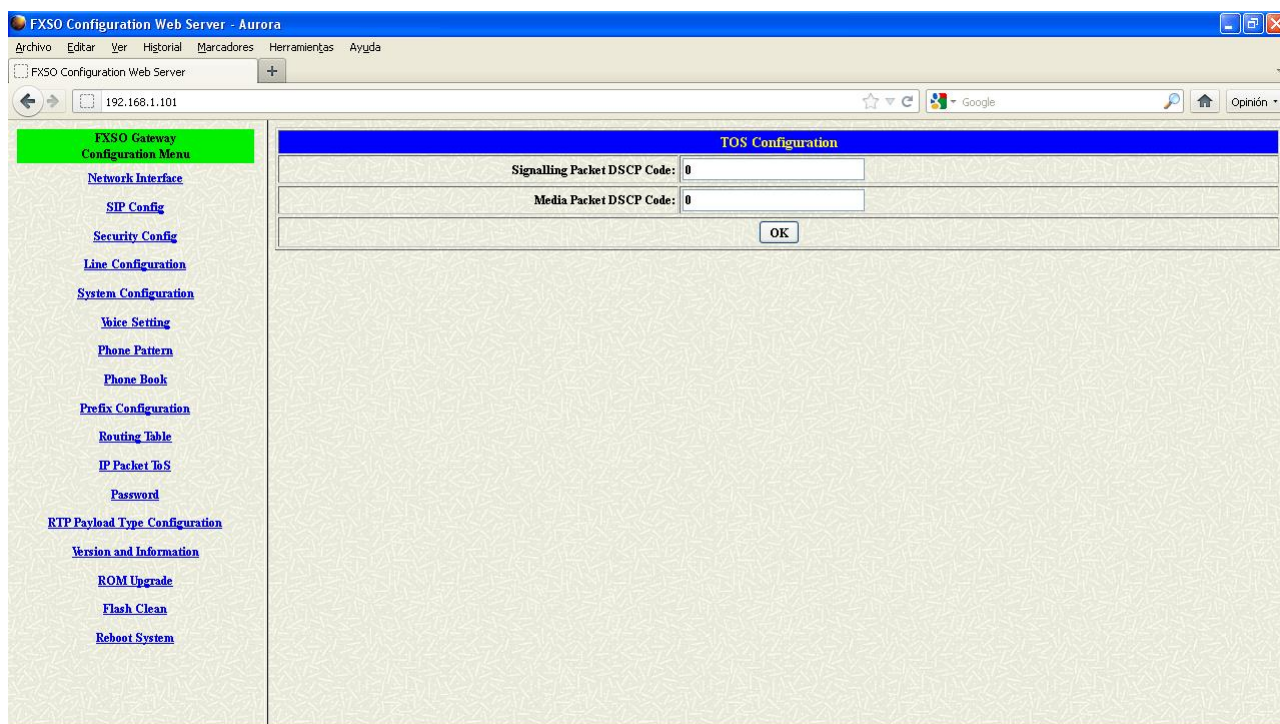
Ilustración 53 - Configuración del tipo de servicio del GW Ip 53 .
